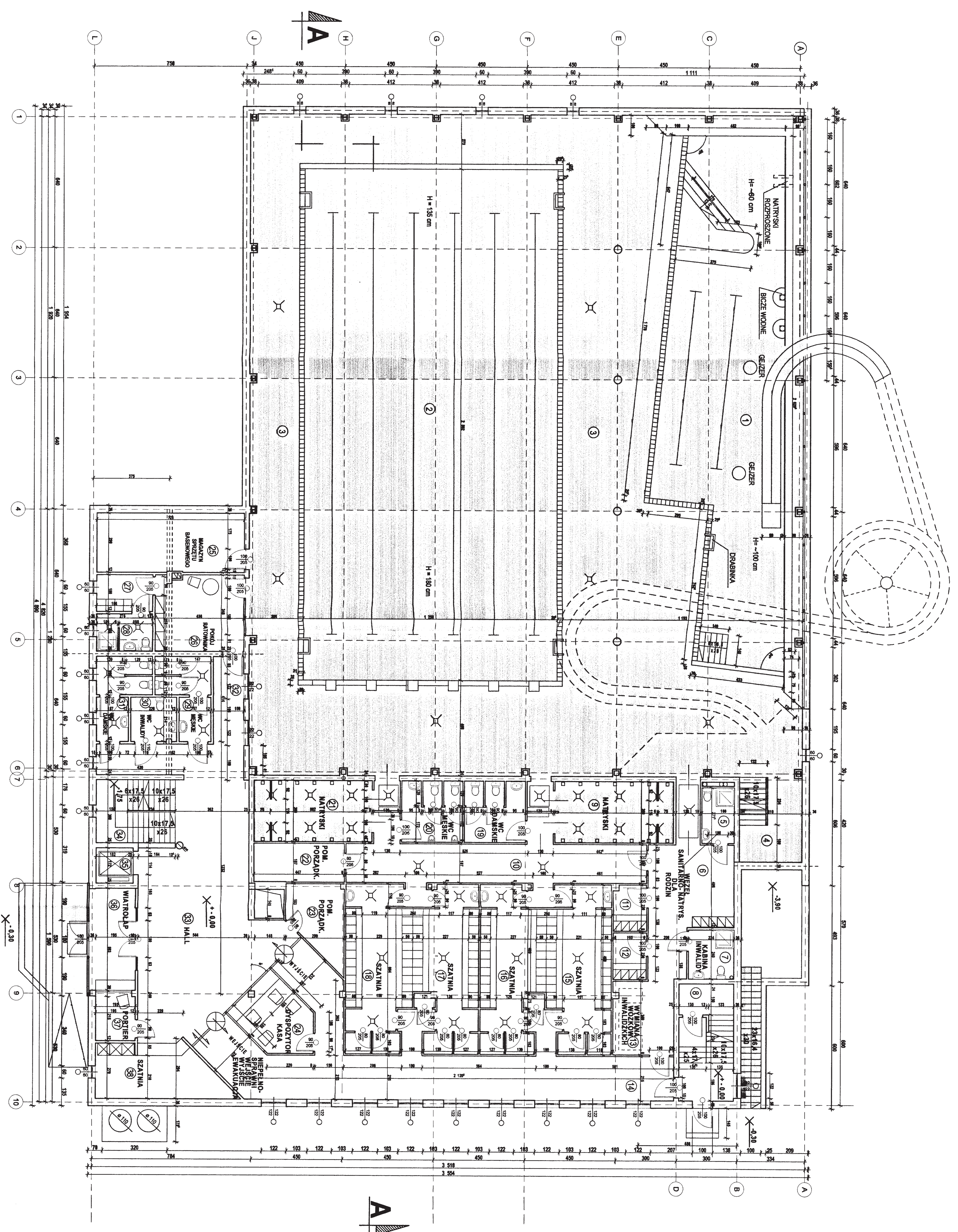
RZUT PARTERU 1:100
